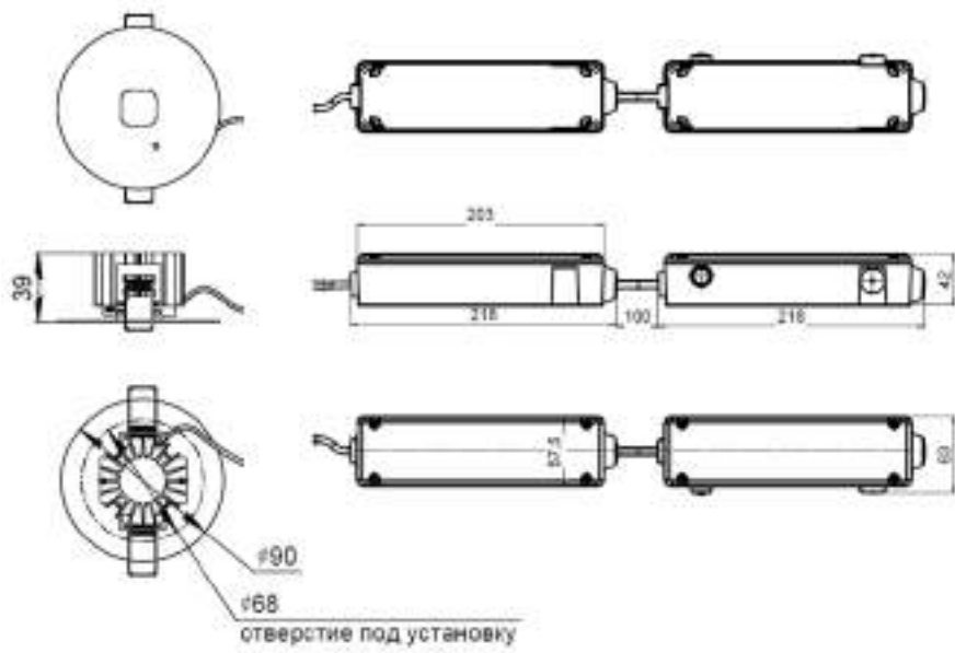
Рис. №3 Аксессуары Стакан потолочный BS-SP-1
